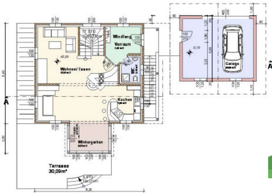
ERDGESCHOSS
