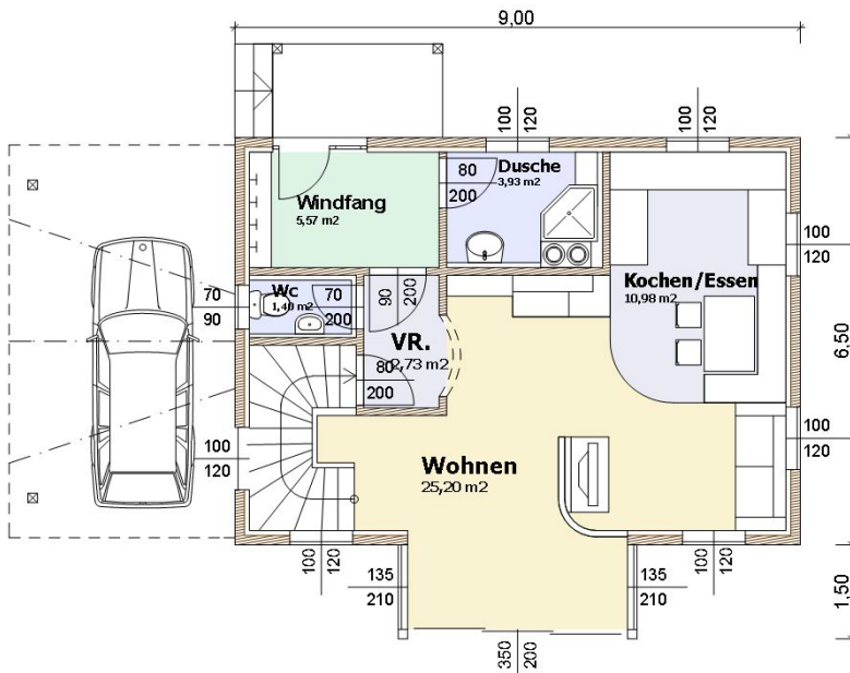
ERDGESCHOSS
