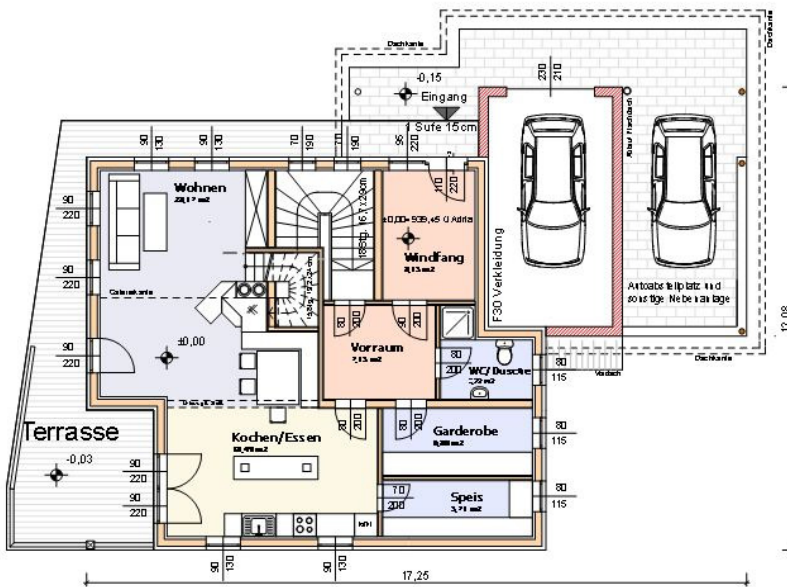
ERDGESCHOSS
