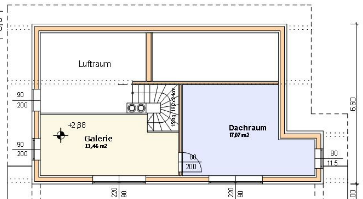
OBERGESCHOSS
