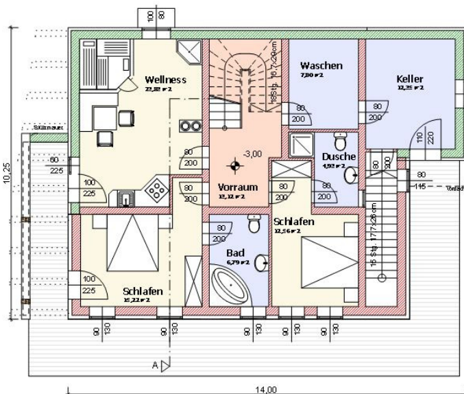
KELLER
