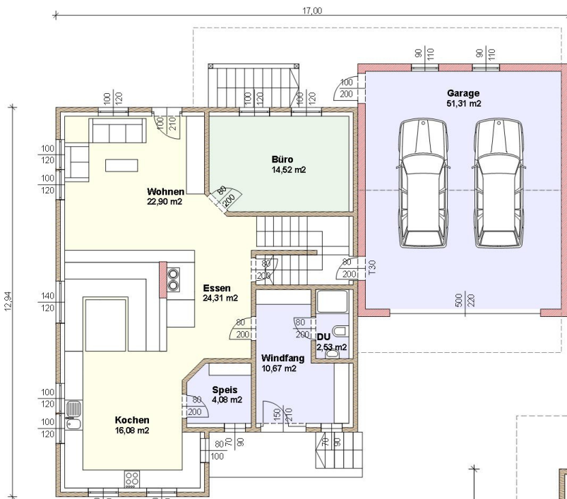
ERDGESCHOSS
